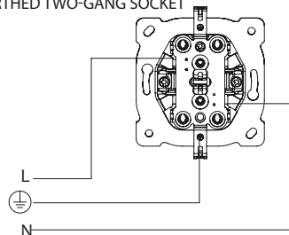
СХЕМА ПІДКЛЮЧЕННЯ Connection Scheme
