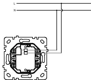
СХЕМА ПІДКЛЮЧЕННЯ Connection Scheme
