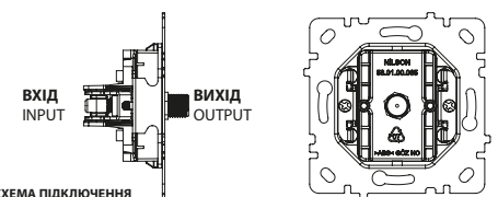
СХЕМА ПІДКЛЮЧЕННЯ Connection Scheme
