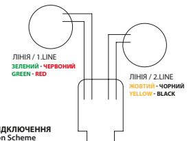
СХЕМА ПІДКЛЮЧЕННЯ Connection Scheme
