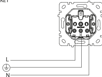
СХЕМА ПІДКЛЮЧЕННЯ Connection Scheme
